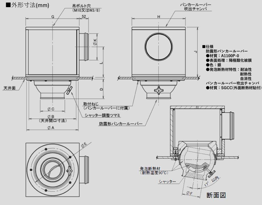
写真は防露型パンカーラーバーとパンカーラーバー吹出チャンバを組み合わせたものです。
